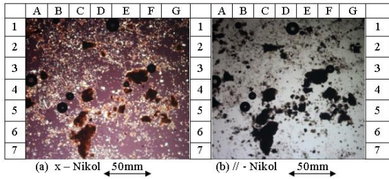
Gambar 21. (a) Sayatan tipis sampel tanah profil 10 lapisan 1 dengan nikel, (b) Sayatan tipis sampel tanah profil 10 lapisan 1 tanpa nikel. biotit (3E), mineral liat (6C), piroxin (5D) dan kuarsa (7D).
