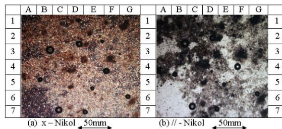
Gambar 6. (a) Sayatan tipis bahan induk rofil 10 dengan nikol, (b) Sayatan tipis bahan induk profil 10 tanpa nikol. biotit (4D), mineral liat (5F) dan kuarsa (7A).
