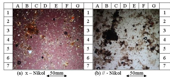
Gambar 22. (a) Sayatan tipis sampel tanah profil 11 lapisan 1 dengan nikel, (b) Sayatan tipis sampel tanah profil 11 lapisan 1 tanpa nikel. Kuarsa (7D), dan biotit (3E)
